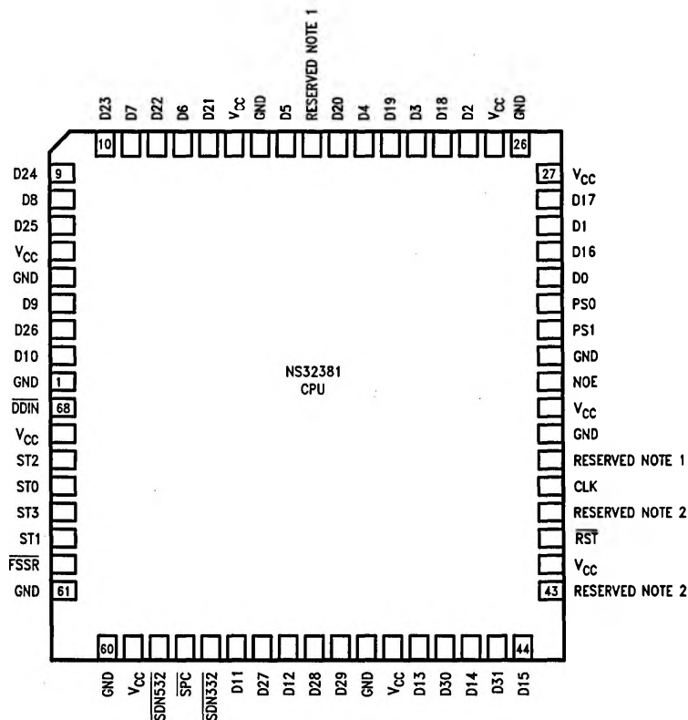
Bottom View Order Number NS32381V-15, NS32381V-20, NS32381V-25 or NS32381V-30 See NS Package Number V68
