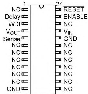
SO-24L
